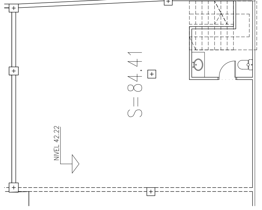
PLANTA SÓTANO
